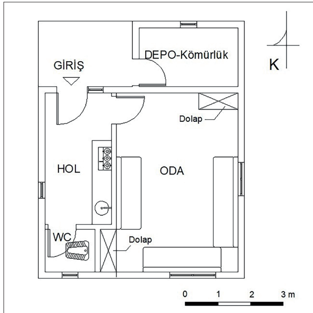
Şekil 6. Yahyaların odası zemin kat planı (Plan yazar tarafından çizilmiştir) / Ground floor plan of Yahya's chamber (The plan was drawn by the author).
