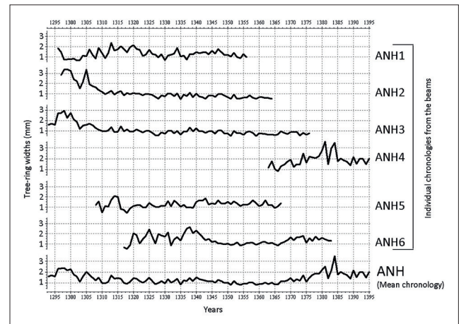
Figure 3. The individual chronologies from the 6 beam samples and their mean chronology (ANH). / Alınan 6 hatıl örneğinin bireysel kronolojileri ve bunlardan elde edilen ortalama kronoloji (ANH).
